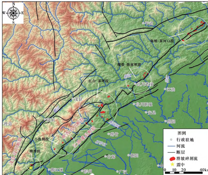
图1 汶川地震典型沟道型滑坡-碎屑流分布图
