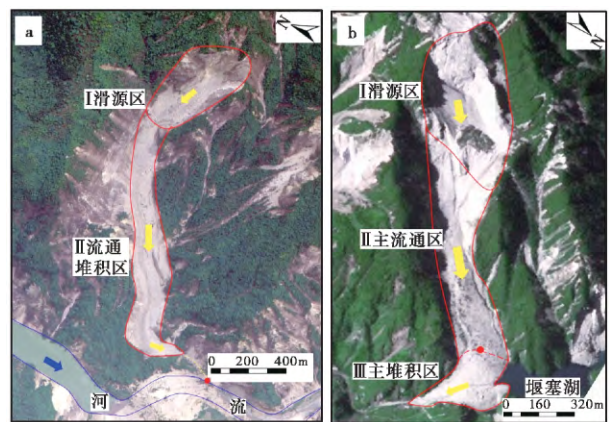
图2 典型沟道型滑坡-碎屑流遥感影像图
