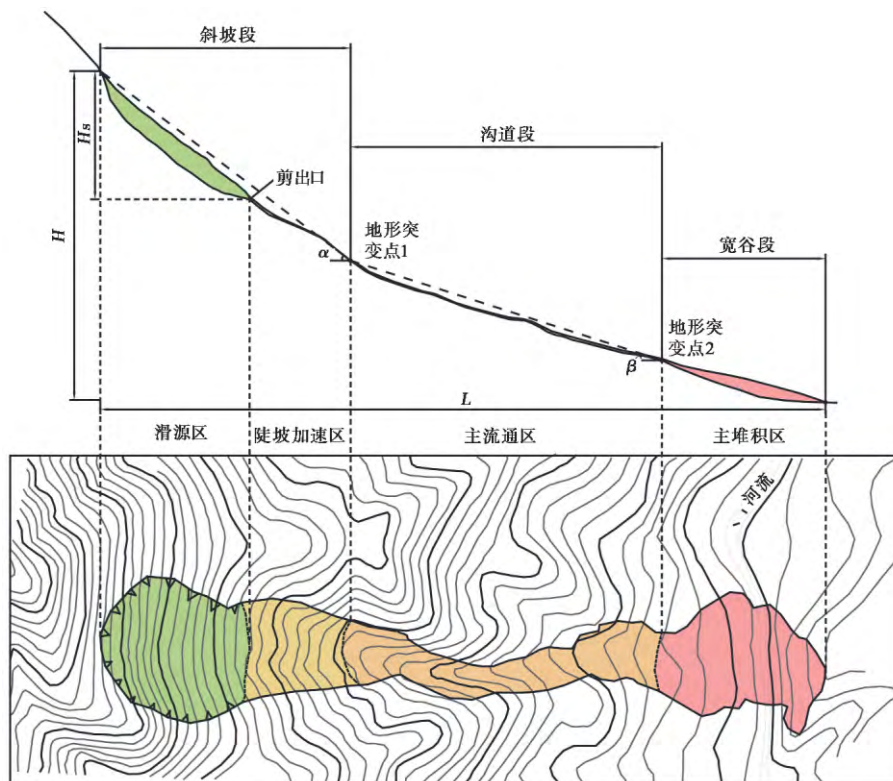
图3 典型沟道型滑坡-碎屑流的示意图
